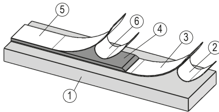
Abb. 1: Montage Magnetband
