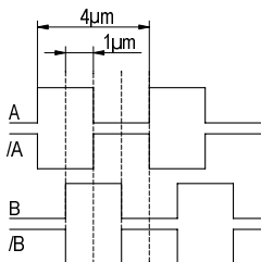
Abb. 2: Ausgabe der Quadratursignale
